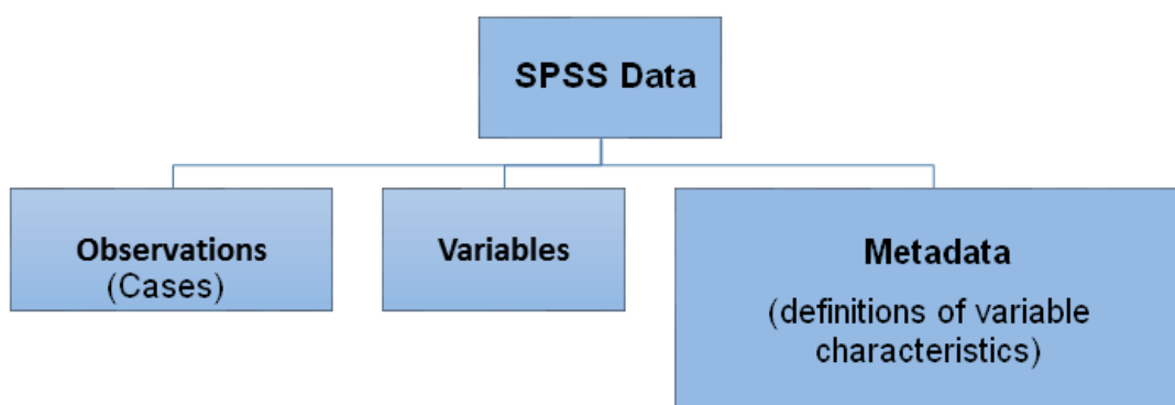
FIGURE 3.2 – Données SPSS.
