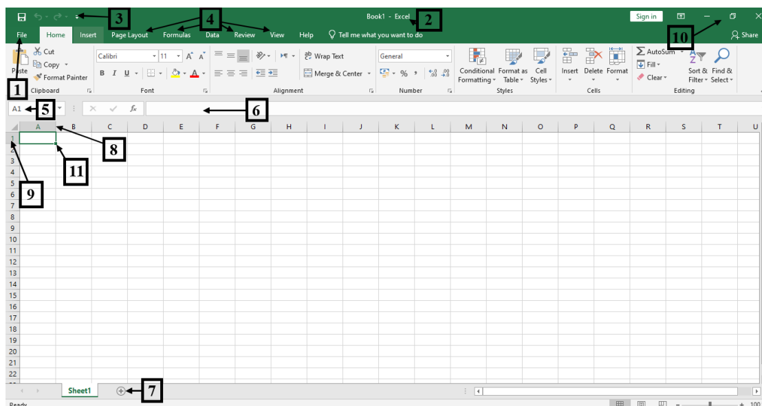
FIGURE 2.1 – Environnement Excel.
